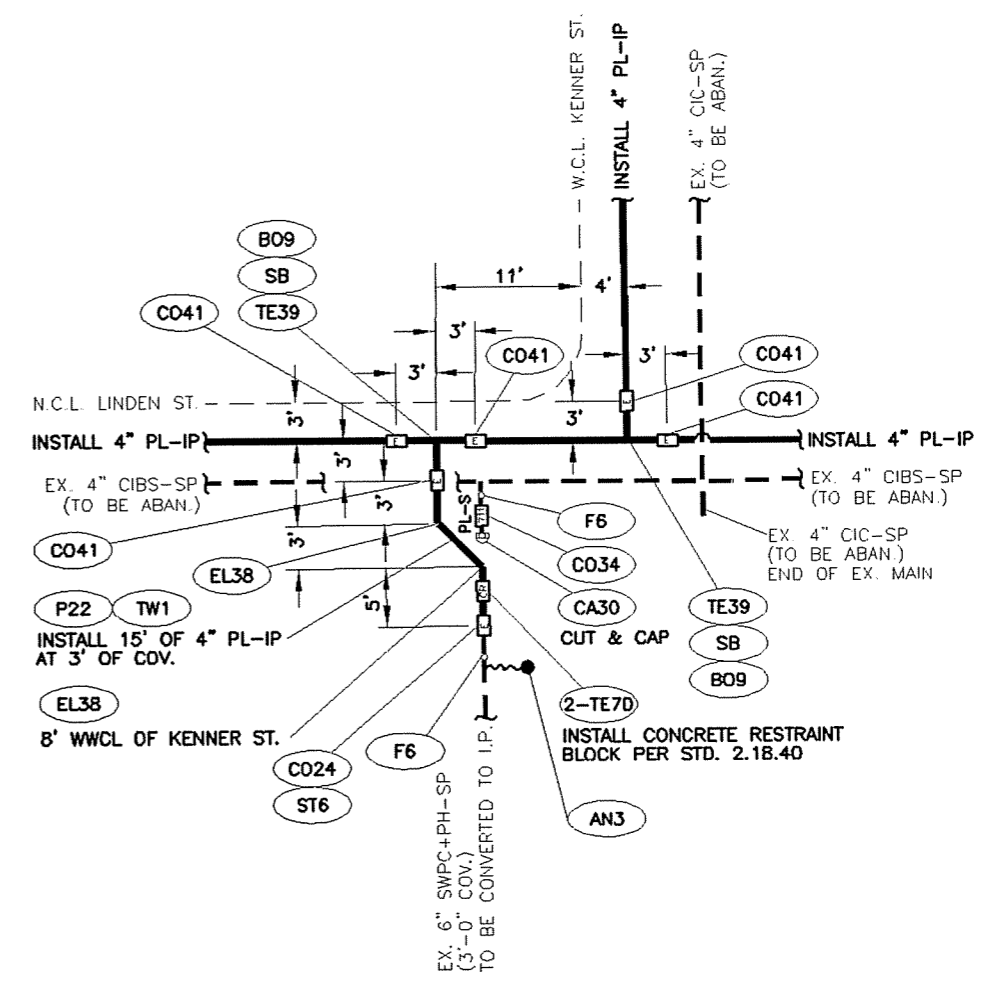
DETAIL "D" (SEE SHEET 9) N.T.S.
