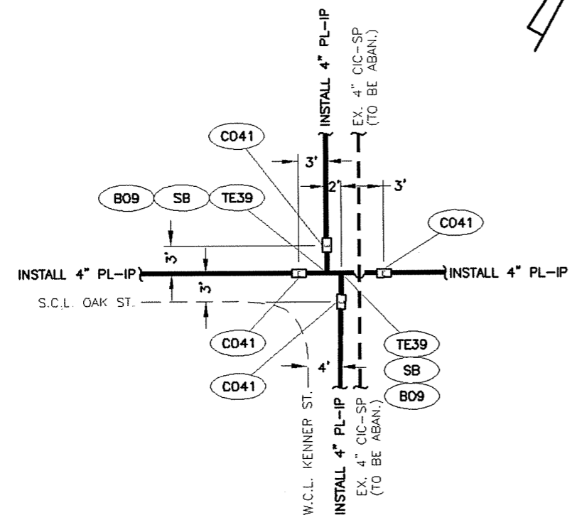
DETAIL "C" (SEE SHEET 9) N.T.S.
