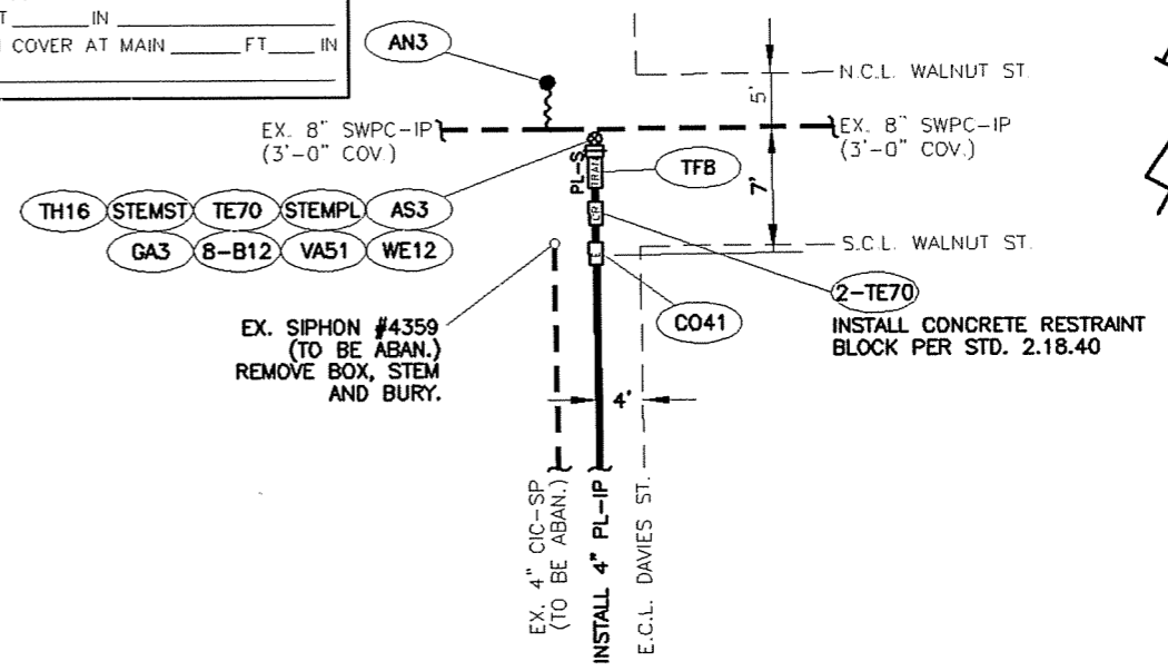
DETAIL "F" (SEE SHEET 11) N.T.S.
