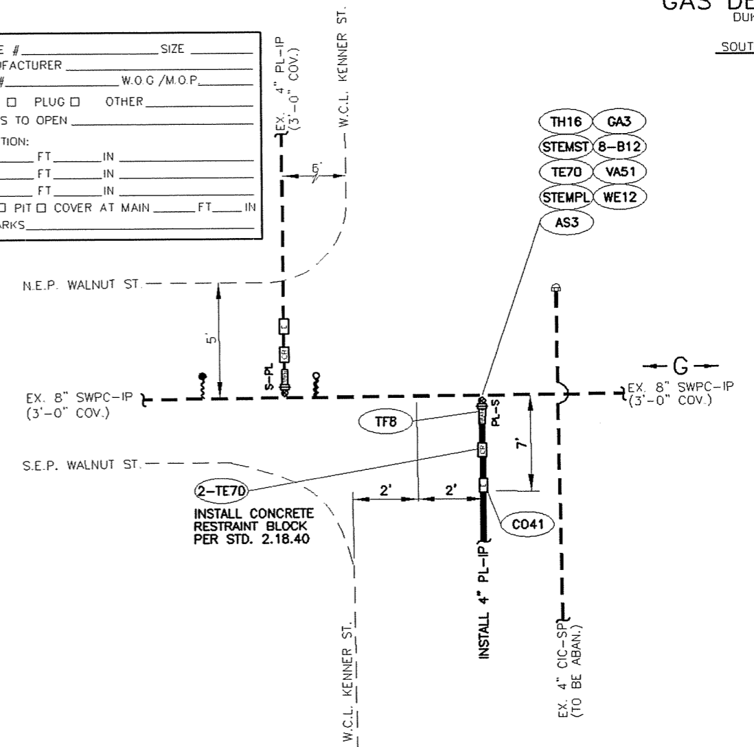
DETAIL "B" (SEE SHEET 8) N.T.S.
