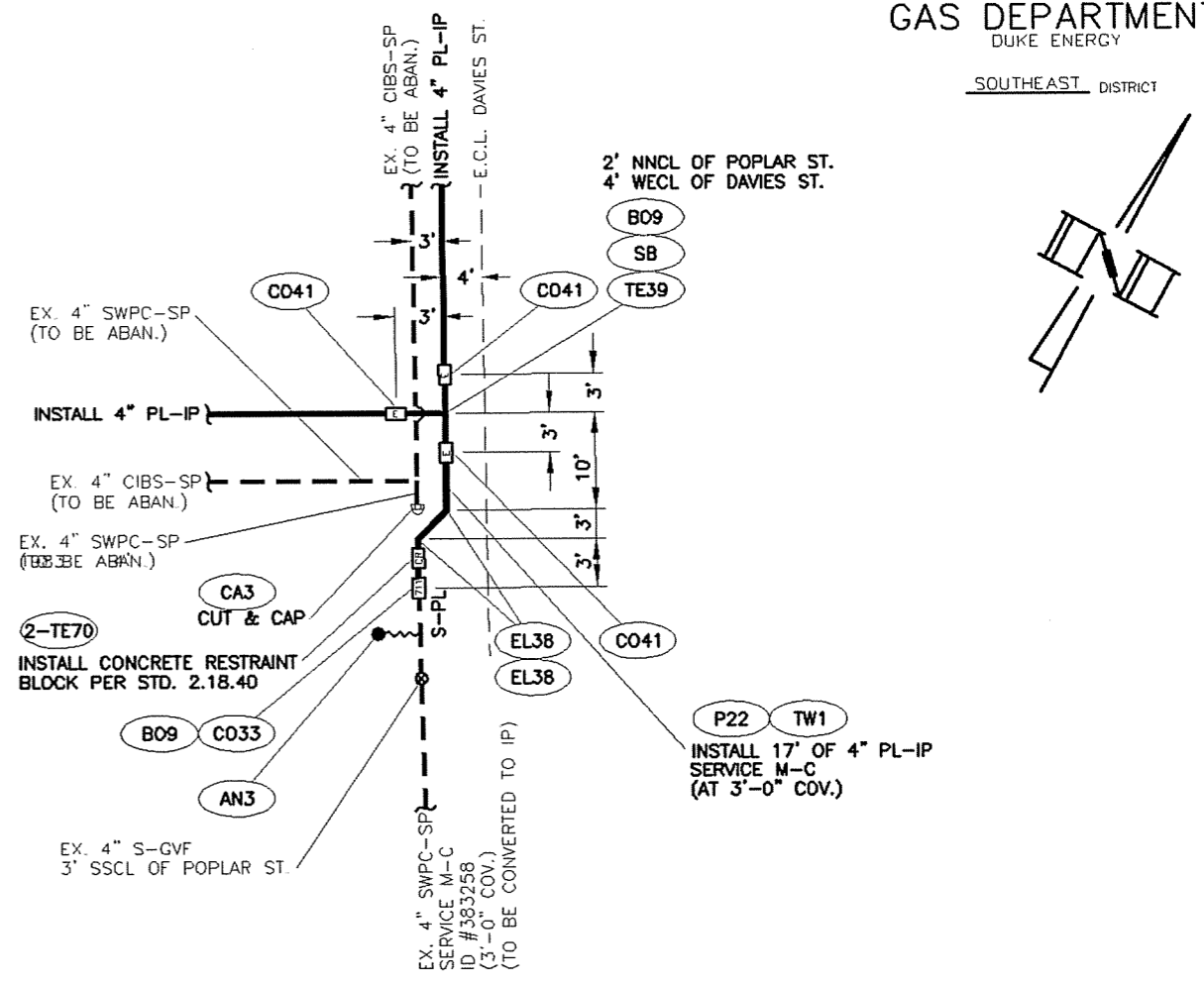
DETAIL "H" (SEE SHEET 13) N.T.S.
