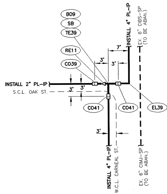
DETAIL "K" (SEE SHEET 15) N.T.S.
