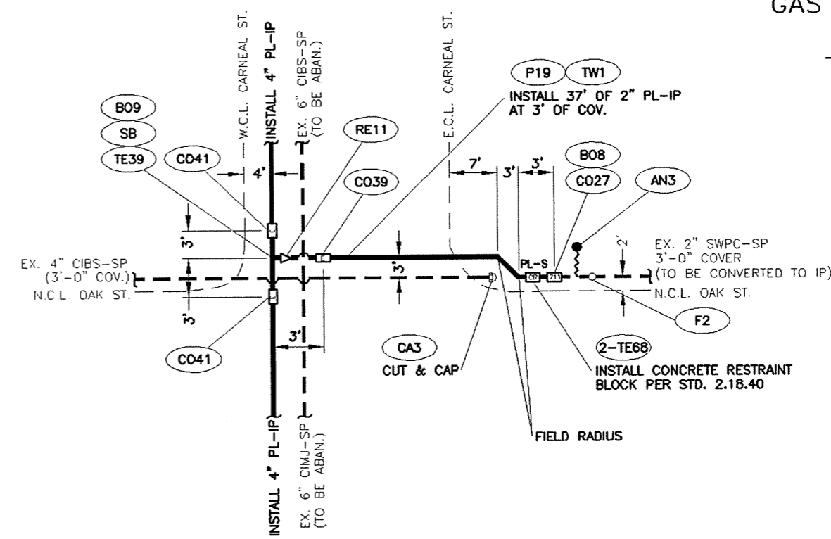
DETAIL "J" (SEE SHEET 15) N.T.S.
