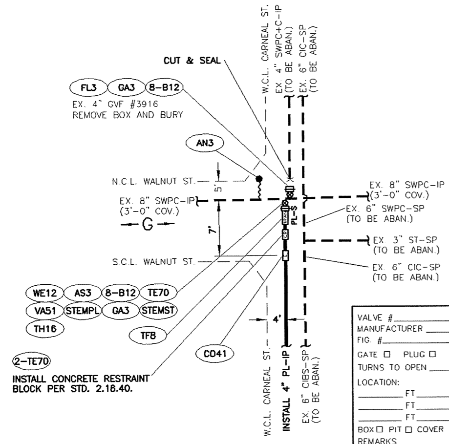
DETAIL "I" (SEE SHEET 14) N.T.S.
