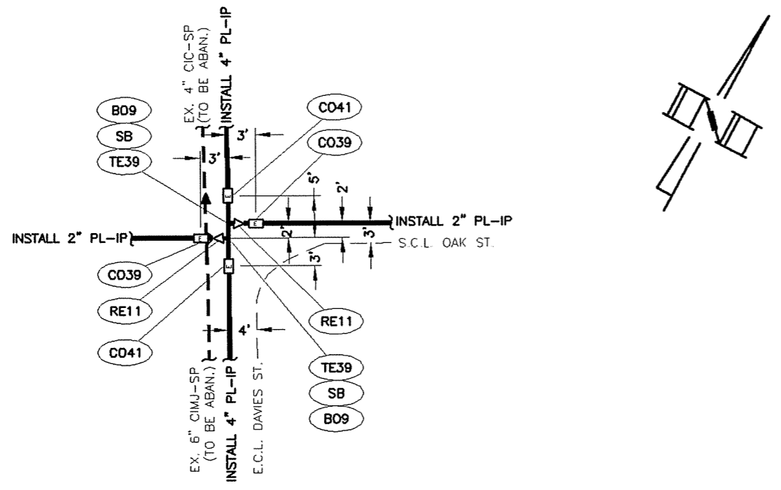
DETAIL "G" (SEE SHEET 12) N.T.S.
